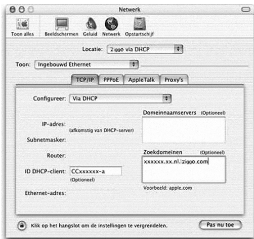
afbeelding 40: TCP/IP instellingen
