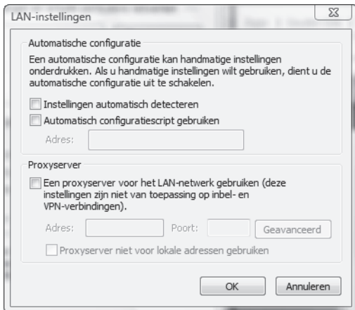
afbeelding 27: LAN-instellingen
