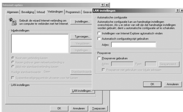
afbeelding 28: Lan-instellingen
