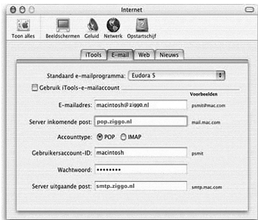
afbeelding 41: E-mailinstellingen
