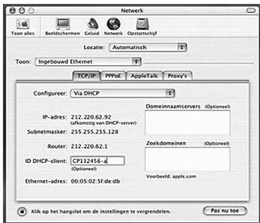
afbeelding 42: TCP/IP instellingen
