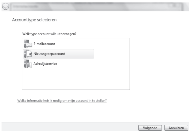
afbeelding 23: Accounttype selecteren
